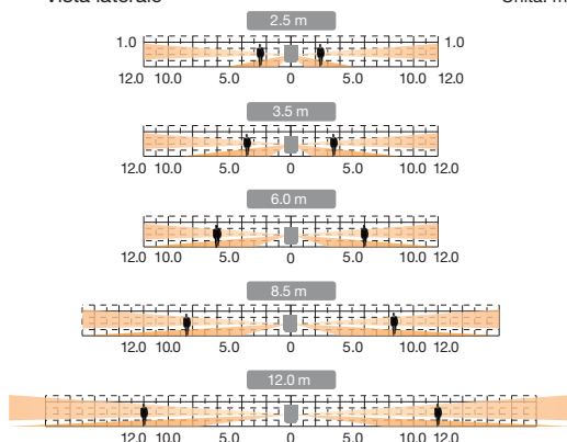
Vista laterale
