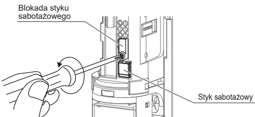
① Poluzuj wkręt.
