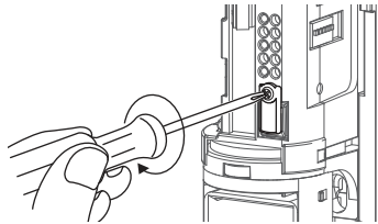
③ Dokręć wkręt blokując styk sabotażowy.
