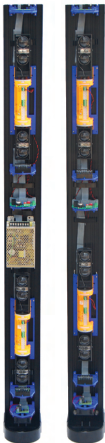
Colonnes 2m pré-montées avec alimentation 220V
