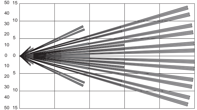
VUE LATÉRALE (Hauteur d'installation 2,3 m (7,6 ft.))
